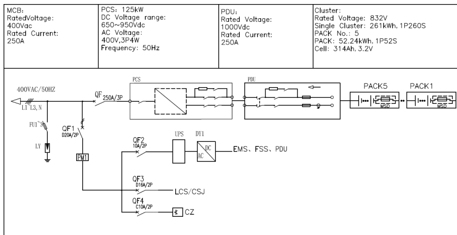
Figura 3-2 Diagrama de la arquitectura eléctrica del sistema
