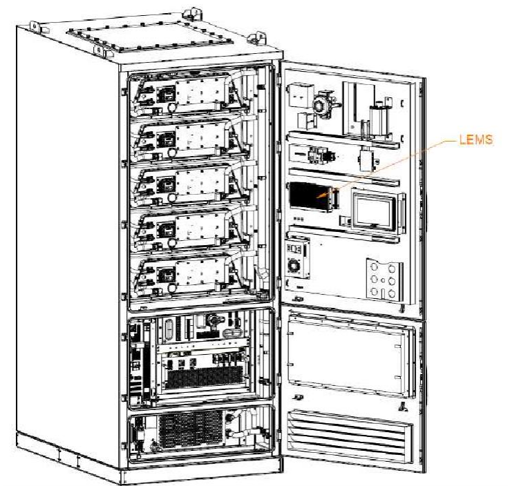
Figura 3-16 Posición del LEMS
