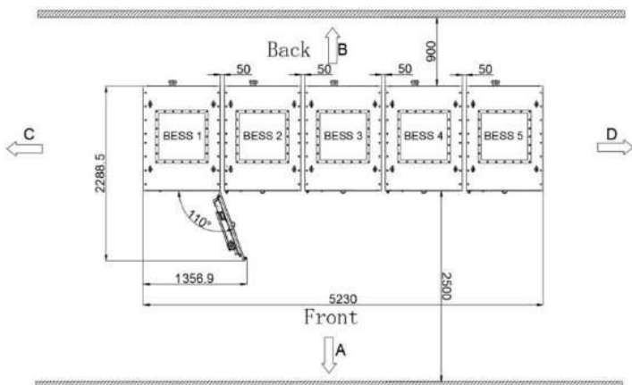
Figura Anexo 4- 3 Esquema 1
