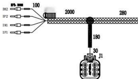
Figura Anexo 4- 23 Cable de comunicación entre ESBCM y ESBMM
