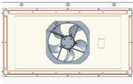
Figura Anexo 6- 49 Orificios de fijación de la placa de montaje del ventilador de refrigeración
