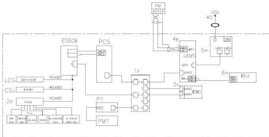
Figura 3-3 Diagrama de la arquitectura de comunicaciones del sistema
