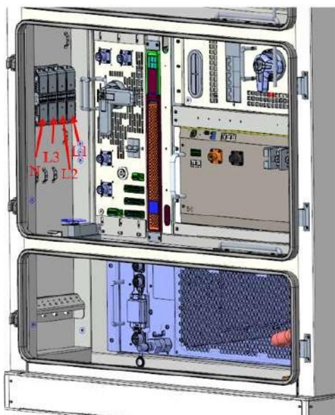
Figura Anexo 6- 1 Cableado del cable de CA
