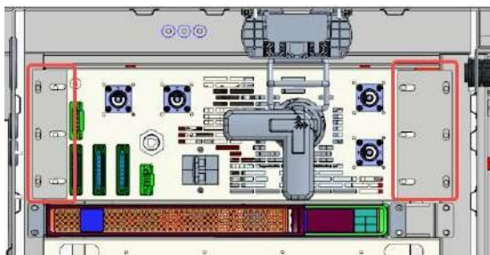
Figura Anexo 6- 47 Tornillos de fijación del panel de la caja de alta tensión
