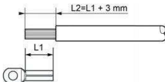
Figura Anexo 6- 3 Longitud de referencia para pelar el cable de tierra
