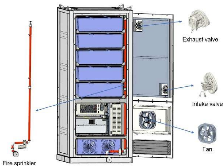
Figura 3-1 Diagrama de anotaciones de los componentes del sistema
