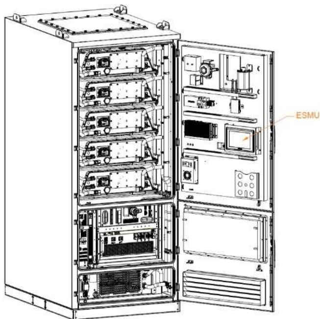
Figura 3-8 Ubicación del ESMU
