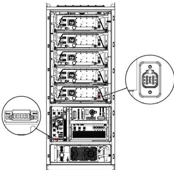
Figura Anexo 4- 25 Conecte el arnés de comunicación/alimentación entre la caja de alta tensión y el paquete de baterías
