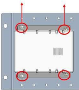
Figura Anexo 6- 32 Retire los tornillos de fijación del detector de gases combustibles
