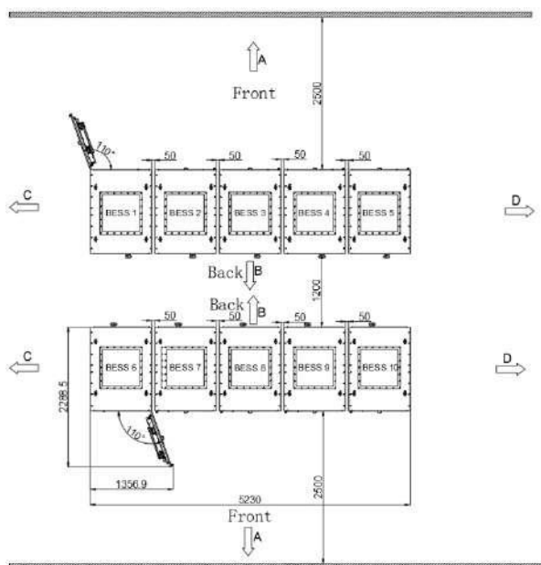
Figura Anexo 4- 5 Esquema del escenario 3
