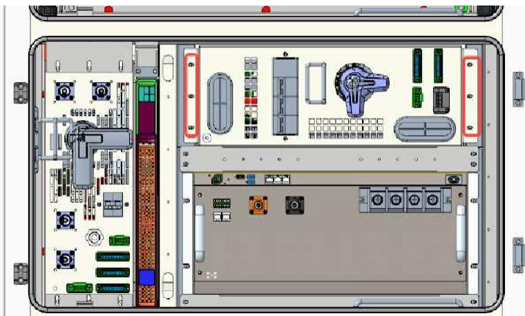
Figura Anexo 6- 42 Placa protectora delantera del conjunto del disyuntor
