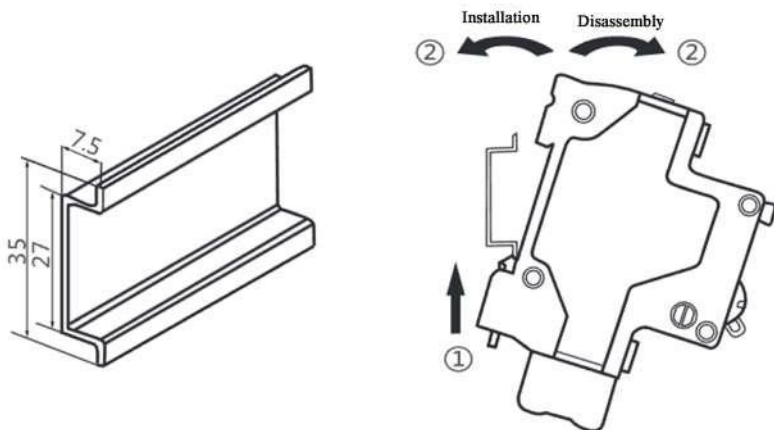
Figura Anexo 6- 52 Sustitución del disyuntor
