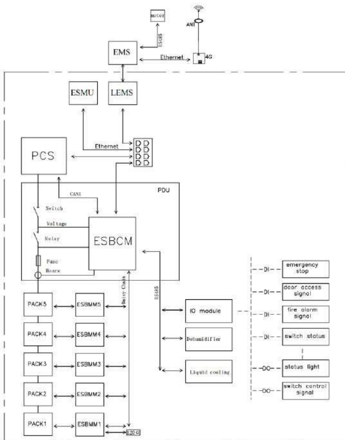
Figura 6-7 Diagrama de la arquitectura del sistema BMS
