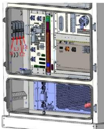
Figura Anexo 6- 8 Conectar el cable de alimentación de salida
