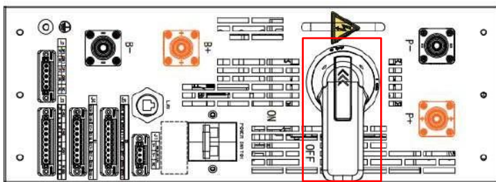
Figura Anexo 4- 19 Disyuntor de la caja de alta tensión en posición «OFF»
