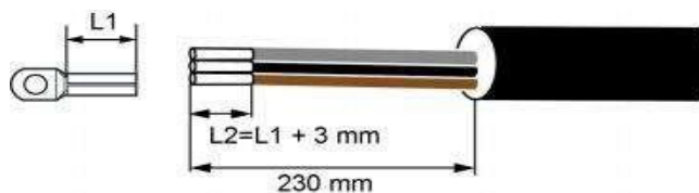
Figura Anexo 6- 5 Longitud de referencia para pelar el cable de alimentación de CA
