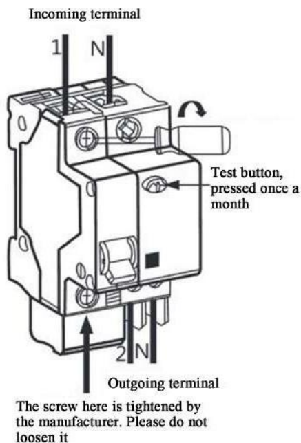
Figura Anexo 6- 51 Disyuntor
