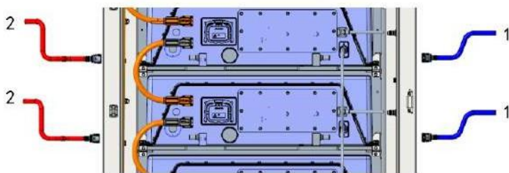
Figura Anexo 4-13 Retire la tubería de refrigerante
