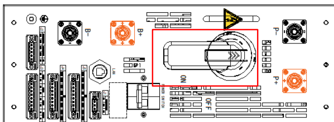
Figura Anexo 4- 28 Disyuntor de la caja de alta tensión en la posición «ON»
