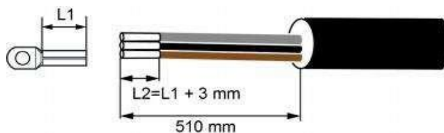
Figura Anexo 6- 4 Longitud de referencia para pelar el cable de alimentación de CA de salida
