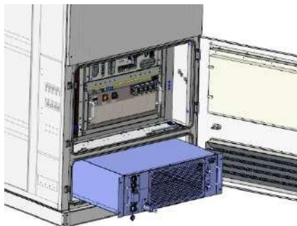
Figura Anexo 6-15 Extraiga la unidad de refrigeración líquida
