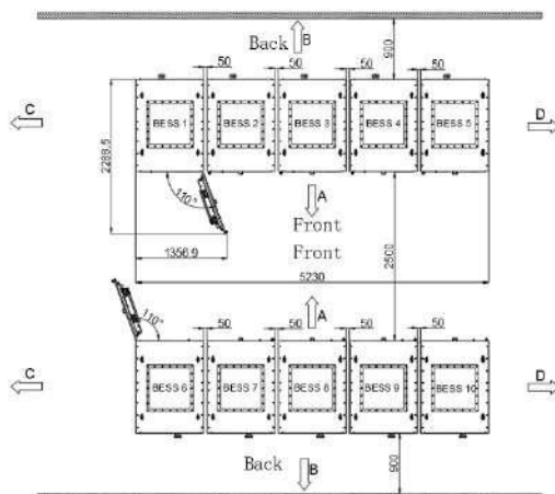
Figura Anexo 4-6 Esquema de distribución 4
