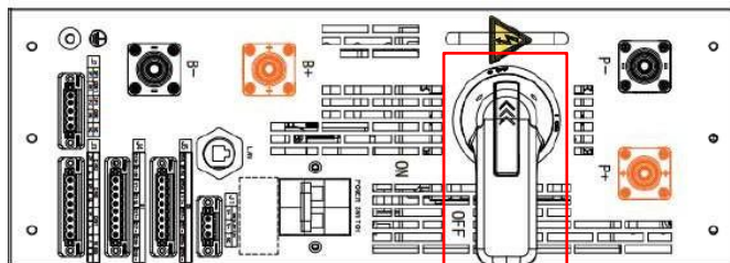
Figura Anexo 4- 27 Disyuntor de la caja de alta tensión en posición «OFF»
