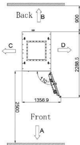
Figura Anexo 4- 3 Esquema 1
