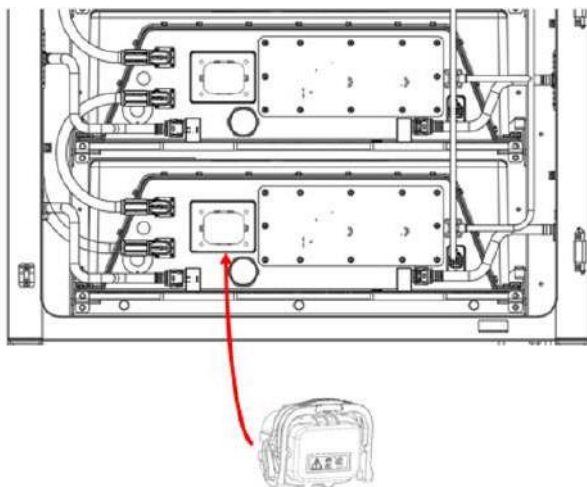
Figura Anexo 4- 33 Posición de instalación del MSD
