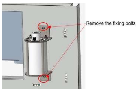
Figura Anexo 6- 35 Retirar el dispositivo extintor
