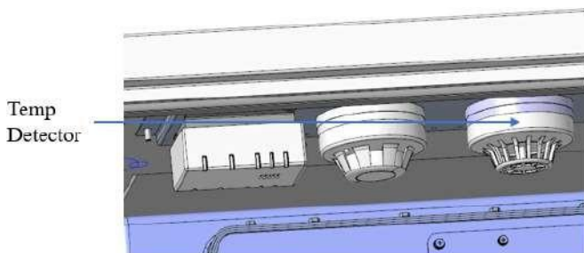
Figura Anexo 6- 29 Posición de instalación del sensor de temperatura
