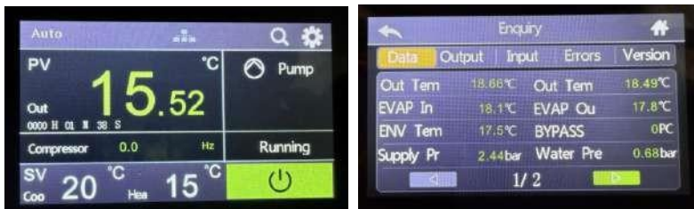
Figura Anexo 6-25 Observe la presión de inyección de líquido
