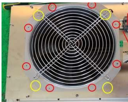
Figura Anexo 6- 50 Orificios de fijación del ventilador de disipación de calor y orificios de fijación del filtro del ventilador
