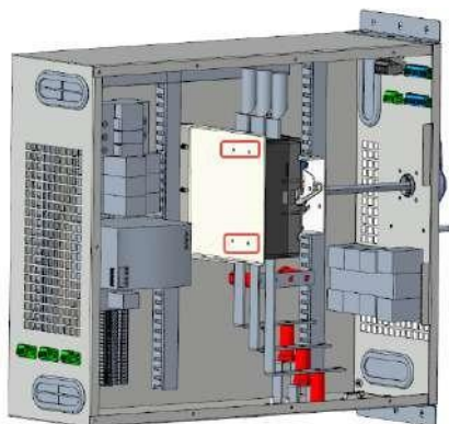
Figura Anexo 6- 45 Retire los pernos de fijación del disyuntor y retire el disyuntor.
